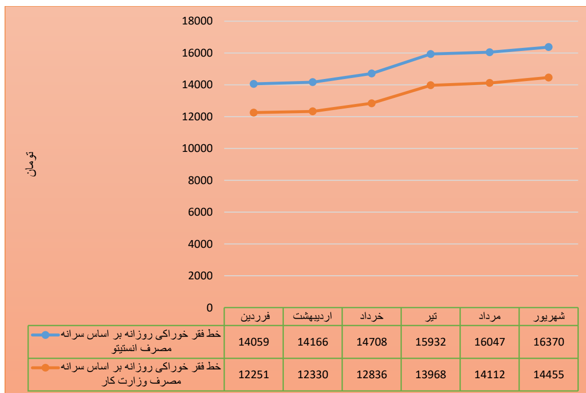
نمودار ۳-۵۹ خط فقر خوراکی روزانه در نقاط روستایی شهرستان قشم
